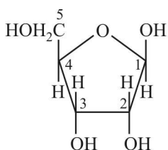
\beta -D-ribose
