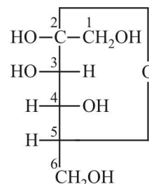
\beta -D-(−)-Fructofuranose
