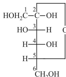
\alpha -D-(−)-Fructofuranose
