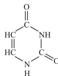
Uracil (U)
